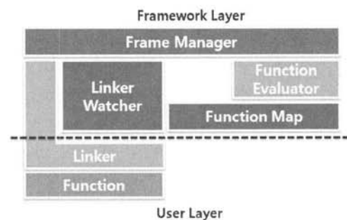
(그림 2) 계층별 프레임워크 구조
