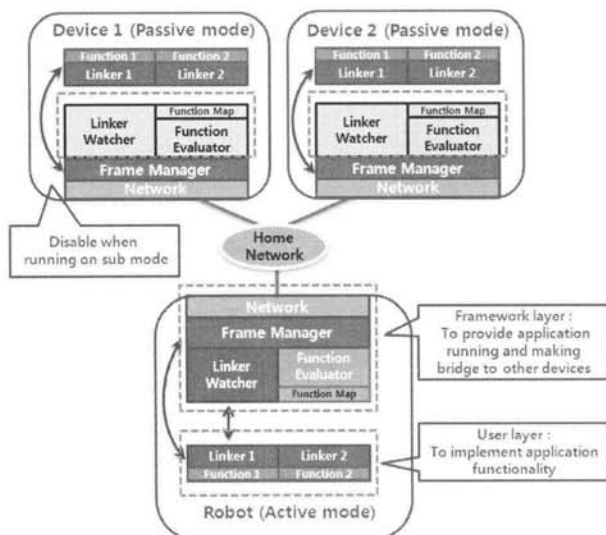
(그림 1) 프레임워크의 구성
