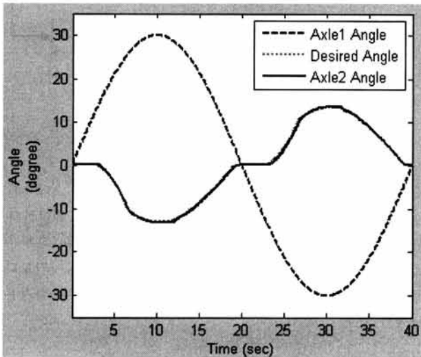
(그림 10) Axle2 performance test
