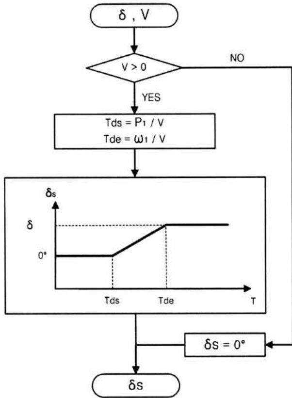
(그림 8) Swing out minimizing algorithm
