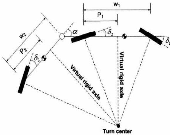
(그림 2) Bicycle Model
