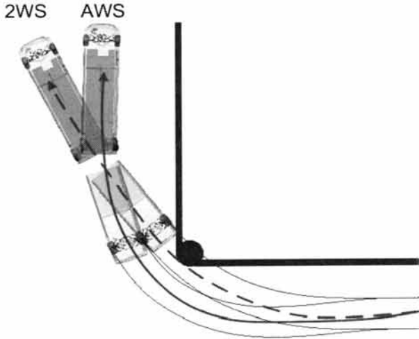
(그림 1) Bi-modal Tram
