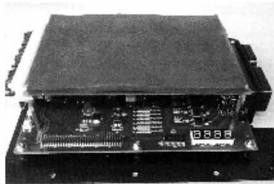
(그림 4) AWS ECU Hardware
