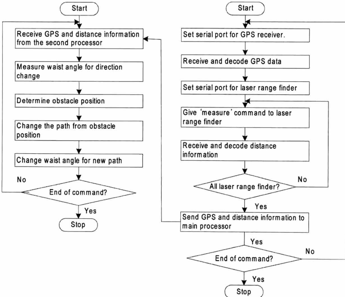
(그림 10) 돌고래 로봇의 흐름도 (Fig. 10) Flowchart for dolphin robot system
