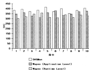
(그림 2) 전체 실행 시간 비교(오류복구포함)
