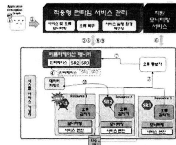
(그림 1) 런타임 서비스 재구성
