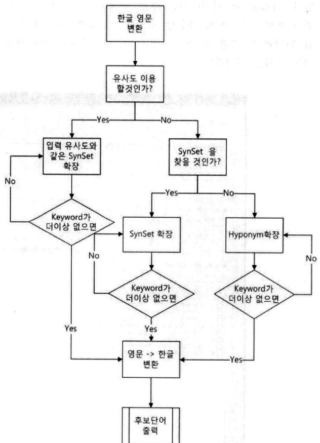
(그림 7) 후보단어 추출 순서도
