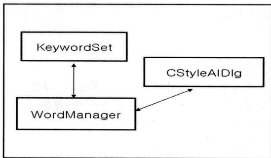
(그림 6) Keyword 추출에 따른 클래스 관계도
