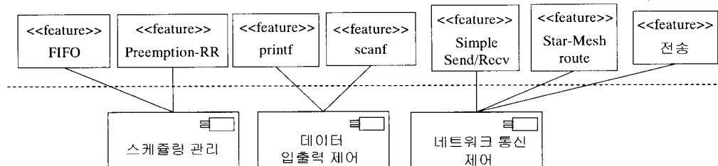
(그림 4) 공통 피쳐와 컴포넌트의 매핑
