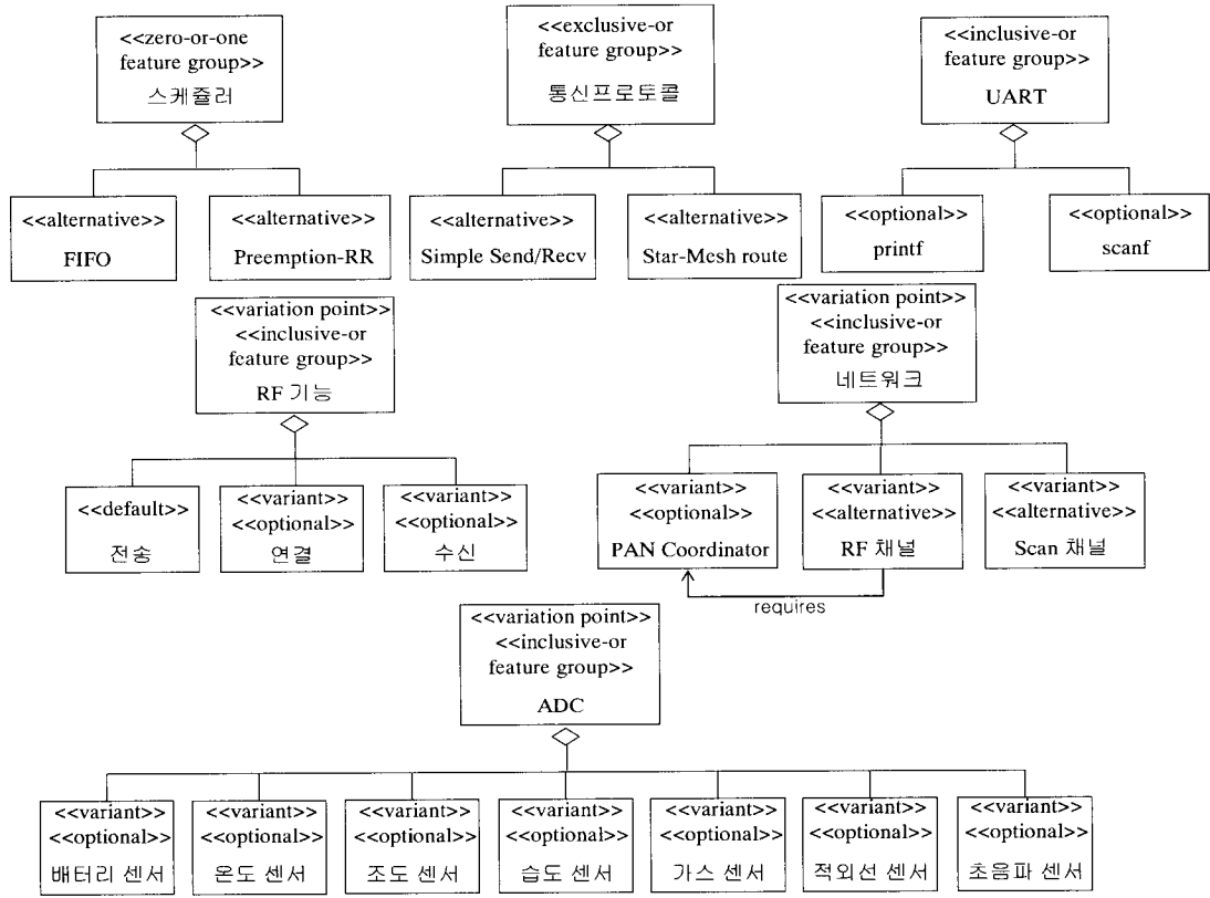
(그림 3) Nano-Qplus 기반의 센서 네트워크 응용 소프트웨어 개발을 위한 가변성 피쳐 모델
