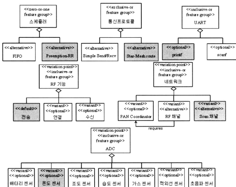
(그림 6) 온도 센서를 위한 응용 소프트웨어의 가변성 피처 모델
