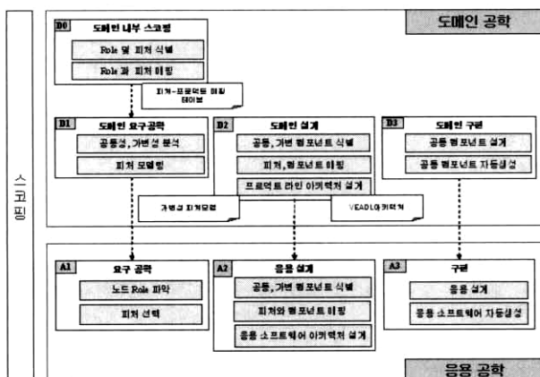
(그림 1) 센서 네트워크 응용 개발 프로세스
