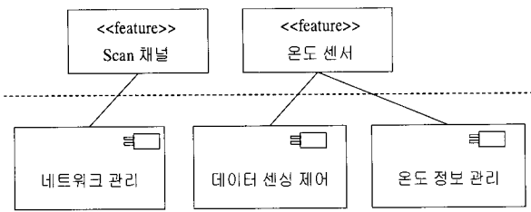
(그림 7) 온도 센서의 응용 소프트웨어를 위한 피처와 컴포넌트의 매핑
