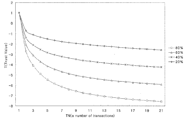
(그림 3) liar의 신뢰 값의 변화
