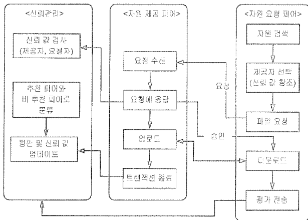
(그림 2) 제안 방안의 동작
