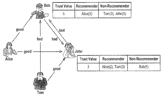
(그림 1) 제안 방안의 동작 예
