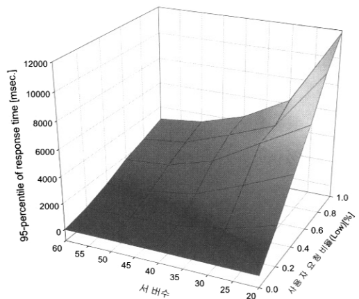
(b) 동적 서버 성능 분할(Low)
