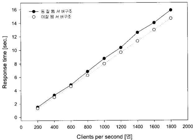
(그림 6) 사용자 도착률에 따른 동질·이질 웹 서버 구조의 응답시간비교
