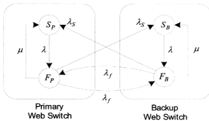
(그림 2) 주-백업 웹 스위치 상태전이도
