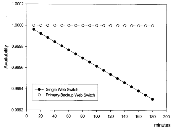
(그림 5) 수리율 변화에 따른 웹 스위치 가용도
