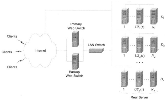
D_i : i 번째 기능 도메인 US_i(t) : 임의의 시간 t 에서 D_i 의 사용자 계층별 요청을 처리하는 서버 구분 경계 값
