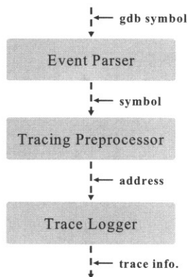
(그림 2) 추적점 엔진의 설계
