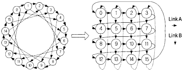
(그림 2) 메쉬 형태로 변환한 건너뛰기 이중 링크 CC-NUMA 시스템 (16 노드, 4 건너뛰기)
