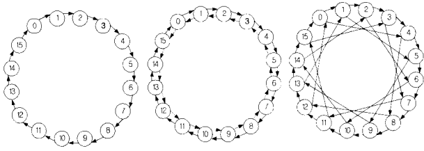
(a) 단일링크 (b) 반대방향 이중 링크 (c) 건너뛰기 이중 링크 (그림 1) 링 구조의 CC-NUMA 시스템 (16 노드)
