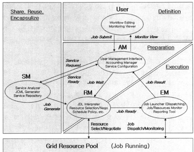
(그림 7) MSSF 시스템 구조
