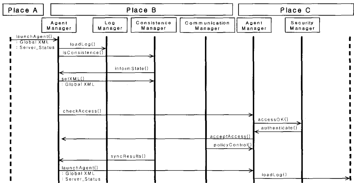
(그림 6) 데이터 동기화 메커니즘
