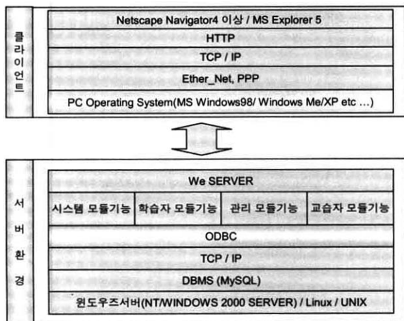
(그림 5) 시스템의 계층구조
