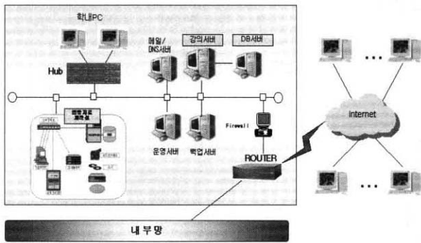
(그림 6) 실험시스템 구성도
