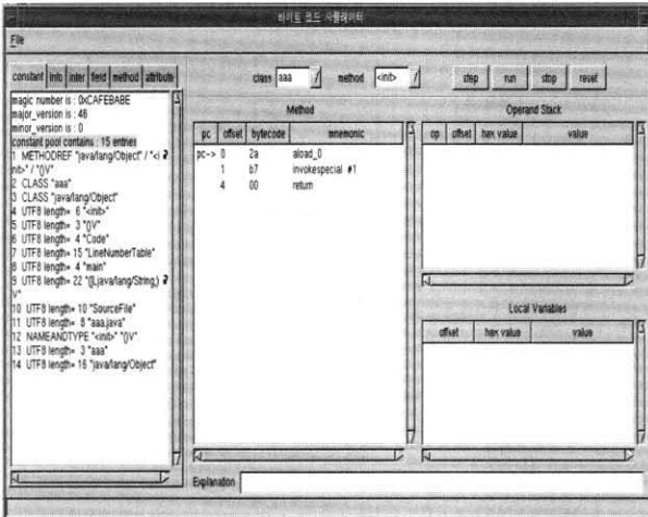
(그림 7) 클래스 파일 정보 표현
