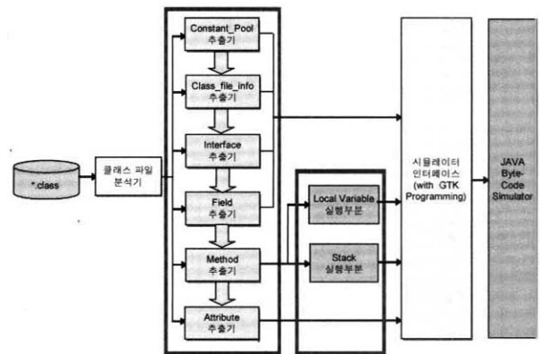
(그림 3) 자바 클래스 파일 실행 분석기 구성
