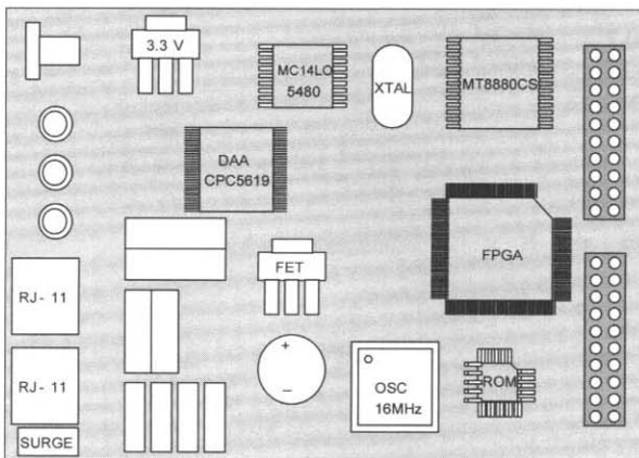
(그림 11) 전화 인터페이스의 구성도
