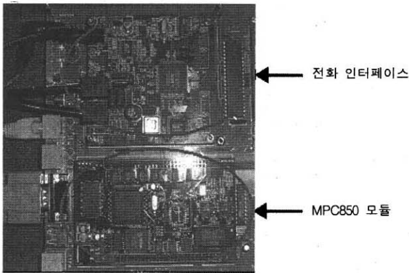
(그림 10) 음성 게이트웨이 설계 사진
