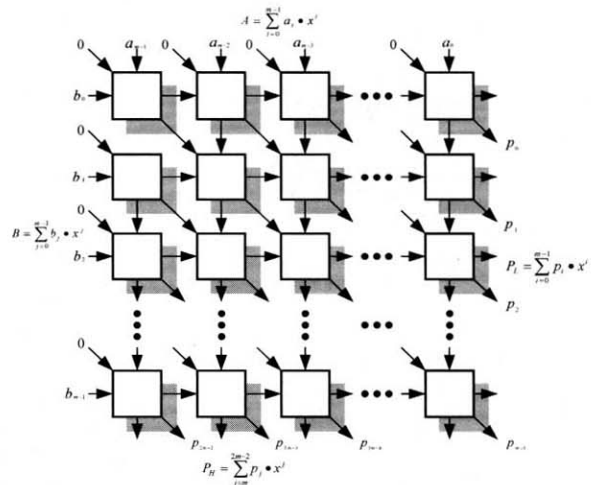
(그림 3) GF(2^m) 상의 승산연산부
