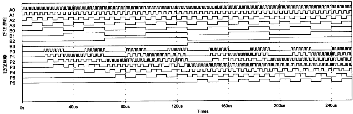
(그림 8) 승산연산부의 시뮬레이션 결과
