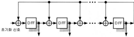
(그림 4) GF(2 m )상의 기약다항식 연산부
