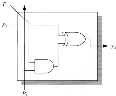
(그림 5) MOD연산부의 기본 셀
