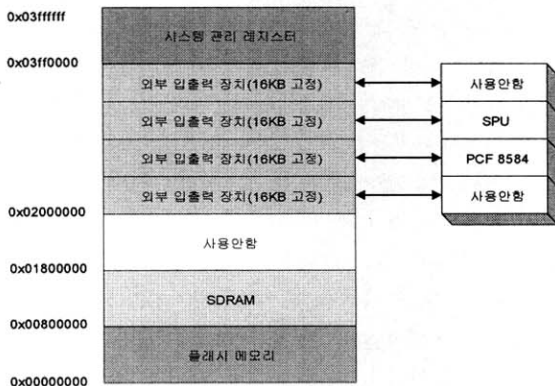
(그림 3) 시스템 메모리 맵
