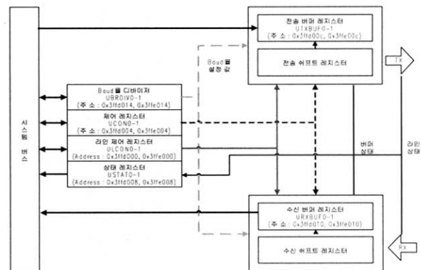
(그림 4) UART 구성 및 컨트롤 블록 다이어그램
