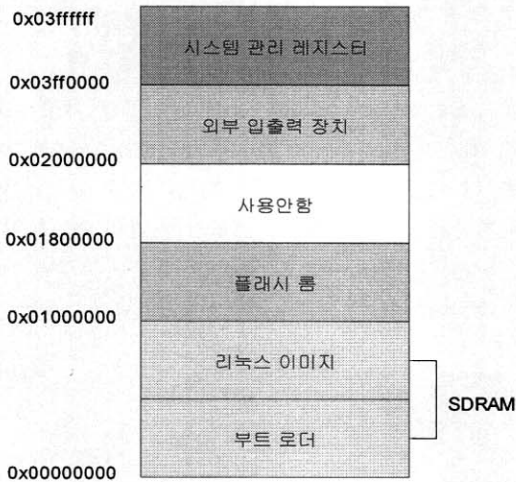
(그림 7) 최종 메모리 맵 상태
