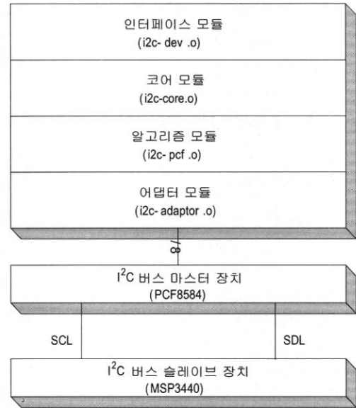
(그림 8) PCF8584 장치 드라이버 구조
