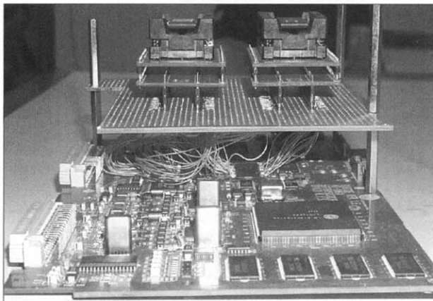
(그림 13) 개발 보드
