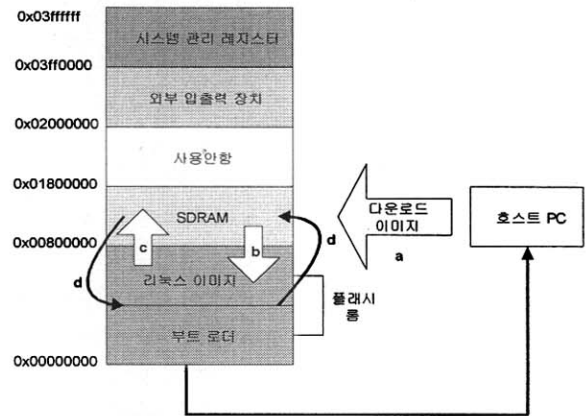
(그림 6) 메모리 맵 설정과정
