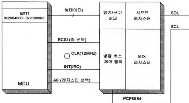
(그림 5) MCU 와 I2C 시리얼 버스 라인의 연결 상태
