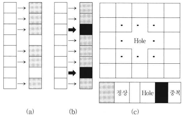
(그림 4) 중복과 Hole
