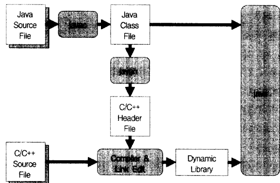
(그림 1) JNI 사용과정
