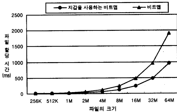
(그림 11) 빈 공간 지갑의 성능
