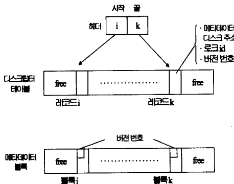
(그림 7) 디스크 저널 자료구조
