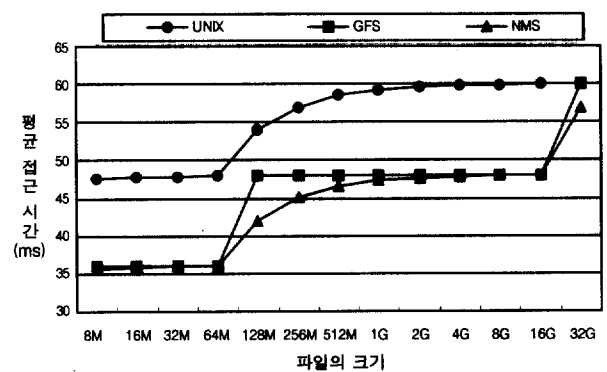
(그림 9) 임의의 블록 접근 시간
