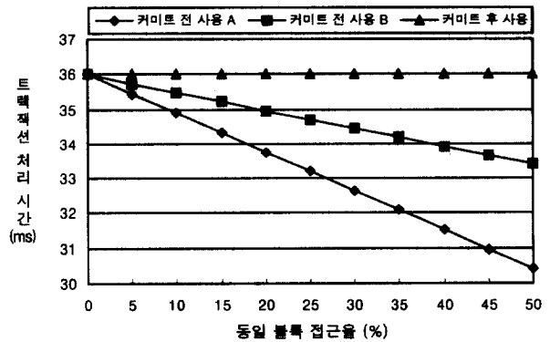
(그림 12) 동일 블록 접근율을 고려한 트랜잭션 처리 시간
