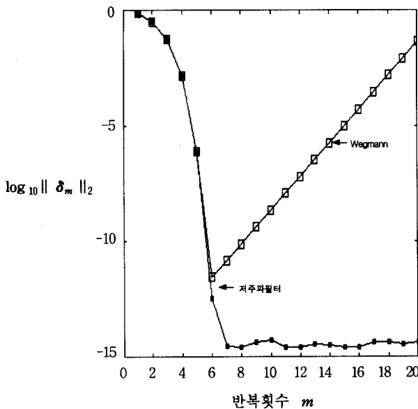
(그림 3) r=0.85 일 때 Wegmann 과 저주파필터 방법에 의한 수정량 비교
