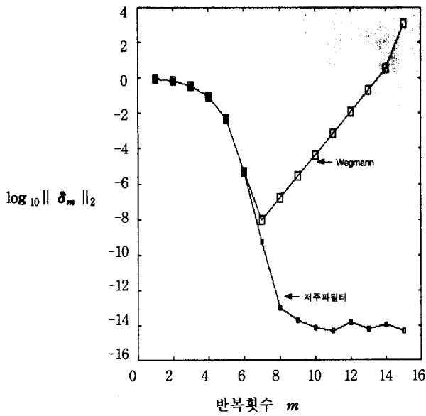
(그림 2) r=0.75 일 때 Wegmann 과 저주파필터 방법에 의한 수정량 비교
