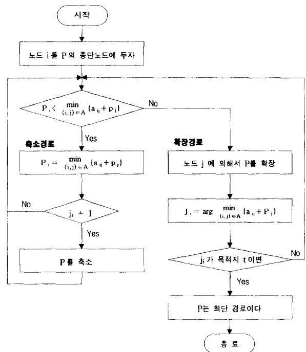
(그림 1) Auction 알고리즘의 전형적 반복
