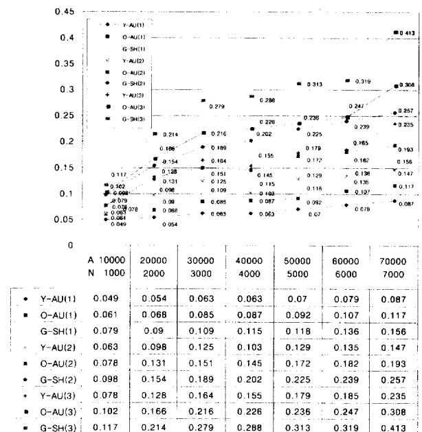
(그림 3) 1개, 2개, 3개 목적지를 가진 경우의 수행결과
