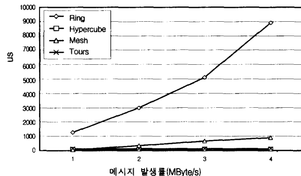
(그림 17) 다중 링크 환경에서 구조별 latency
