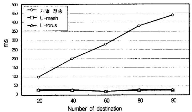
(그림 19) 그물구조에서의 멀티캐스트 latency
