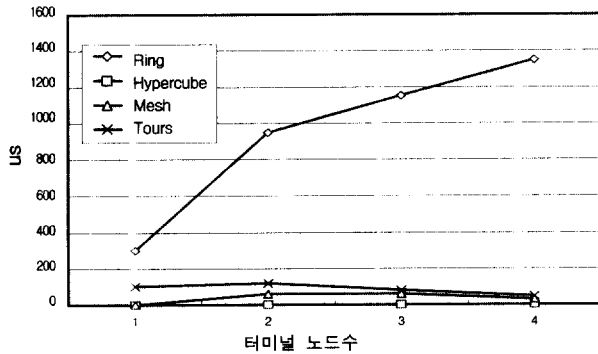
(그림 18) 다중 링크 환경에서 구조별 패킷 정체 시간
