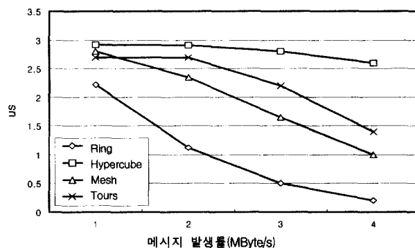
(그림 16) 다중 링크 환경에서 구조별 throughput
