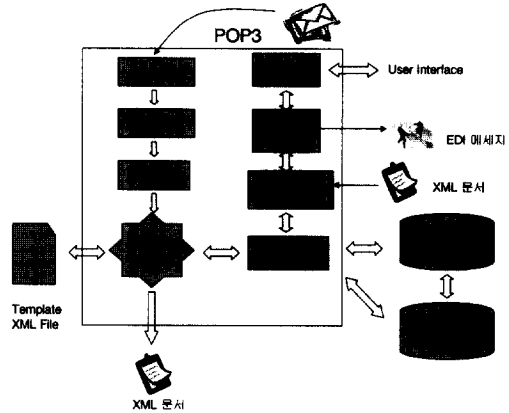
(그림 2.4) 변환기 시스템 세부 구성도
