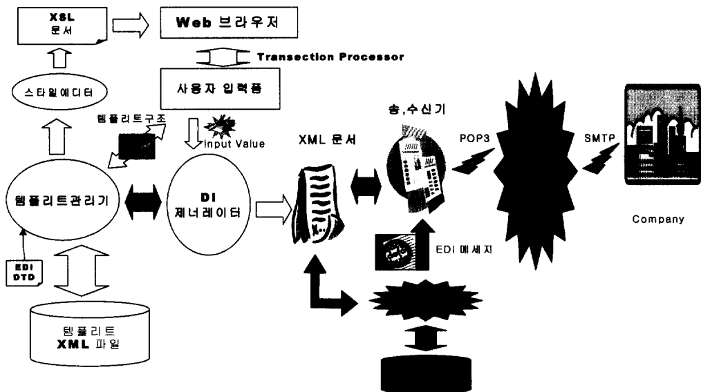
(그림 2.1) 시스템 상세 구성도
