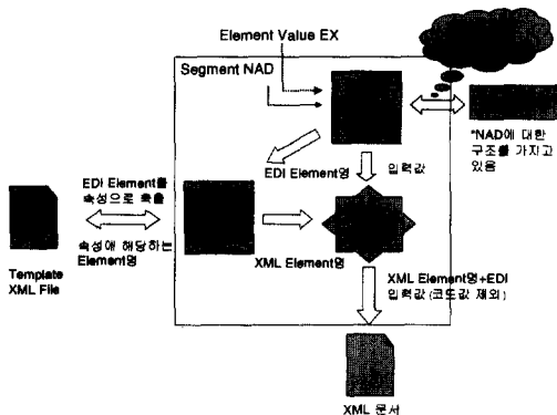
(그림 2.5) XML 문서 생성기
