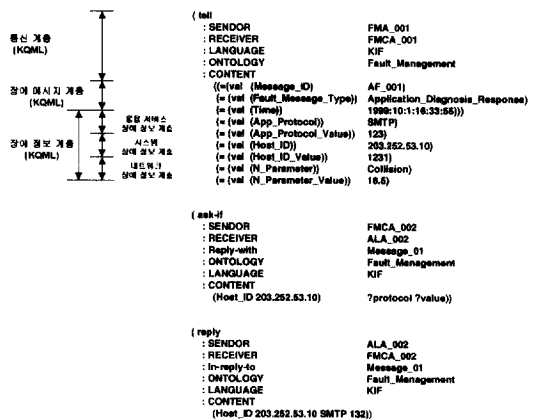
(그림 4) 장애 진단 에이전트 통신 메시지 형식
