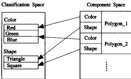
(그림 2) Facet 분류
