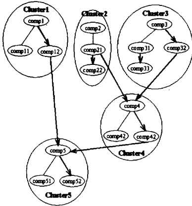
(그림 7) 클래스 라이브러리 클러스터 구성
