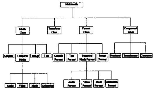
(그림 6) 클래스 라이브러리 Category 구성
