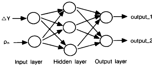
(그림 2) I-프레임 사이의 장면전환 가능성 검출을 위한 신경망 구조
