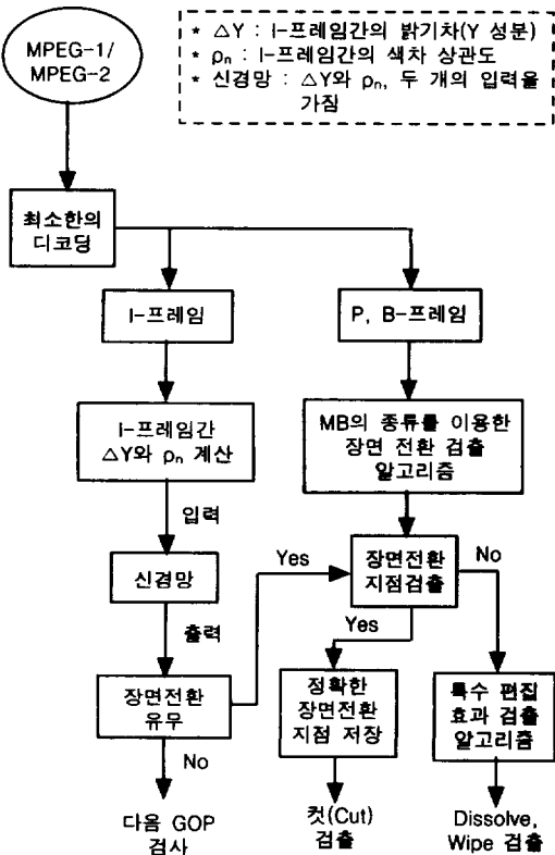
(그림 1) 제안한 계층적인 컷 검출 알고리즘의 흐름도
