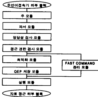
(그림 2) SQL 처리기의 모듈 구조
