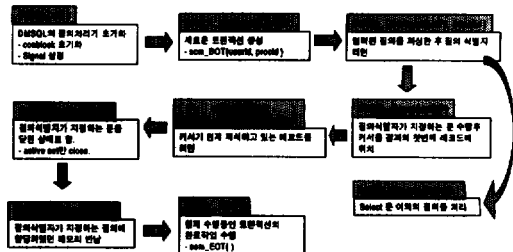
(그림 5) DMSQL Interface Function Flow
