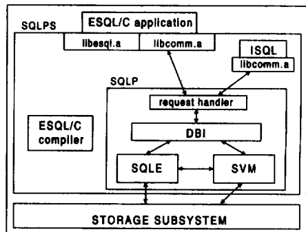
(그림 3) SQLPS의 전체 구조
