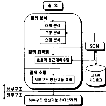
(그림 4) 질의 처리기의 전체 구성
