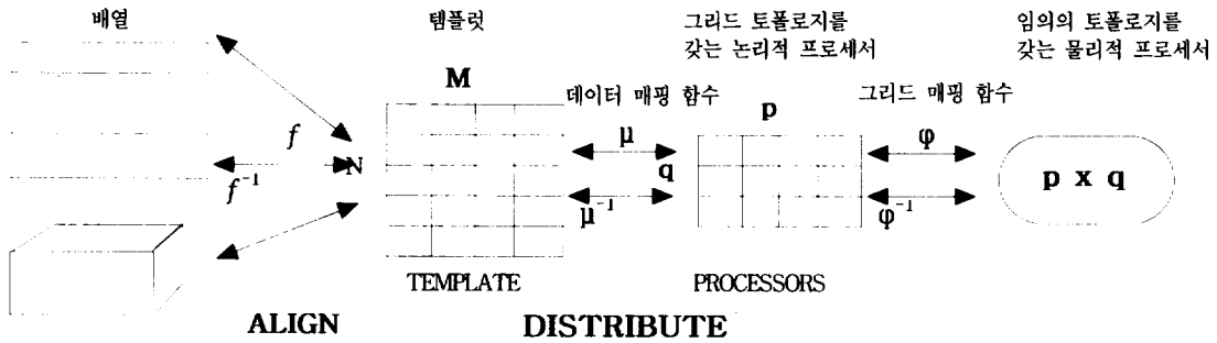
(그림 1) HPF의 데이터 매핑 모델 (Fig. 1) Data mapping model For HPF
