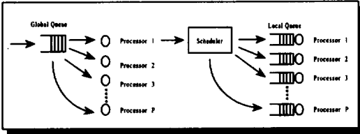
(그림 2) Task Allocation Methods
