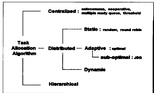
(그림 1) 타스크 할당 알고리즘의 분류 (Fig. 1) Classification of Task Allocation Algorithms
