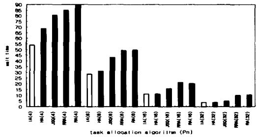
(c) \lambda = 5 일 때
