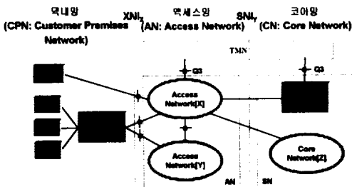
(그림 1) 액세스망 참조 모델 (Fig. 1) Access Network Reference Model
