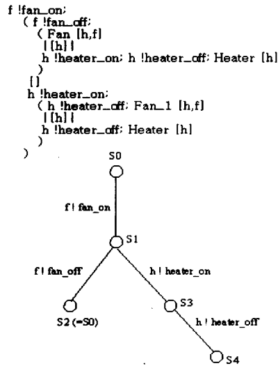
(그림 3) LOTOS 확장 트리 (Fig. 3) Expansion Tree of LOTOS Spec.
