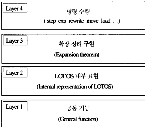
(그림 6) LOLA 라이브러리의 계층 구조 (Fig. 6) Layers of LOLA Library
