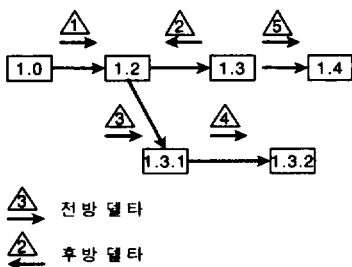
(그림 1) 전·후방 델타에 의한 버전들
