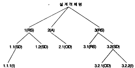
(그림 7) 전역 버전 관리 트리 (Fig. 7) A war zone version management tree
