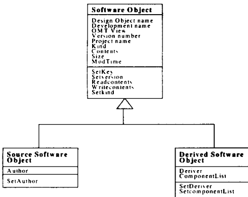
(그림 4) 소프트웨어 객체에 대한 클래스 정의 (Fig. 4) Class definition for software objects
