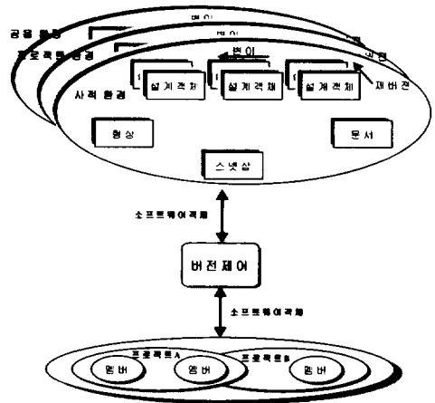
(그림 3) 다른 환경에서 소프트웨어 객체 관리 (Fig. 3) Software objects and their management in different contexts
