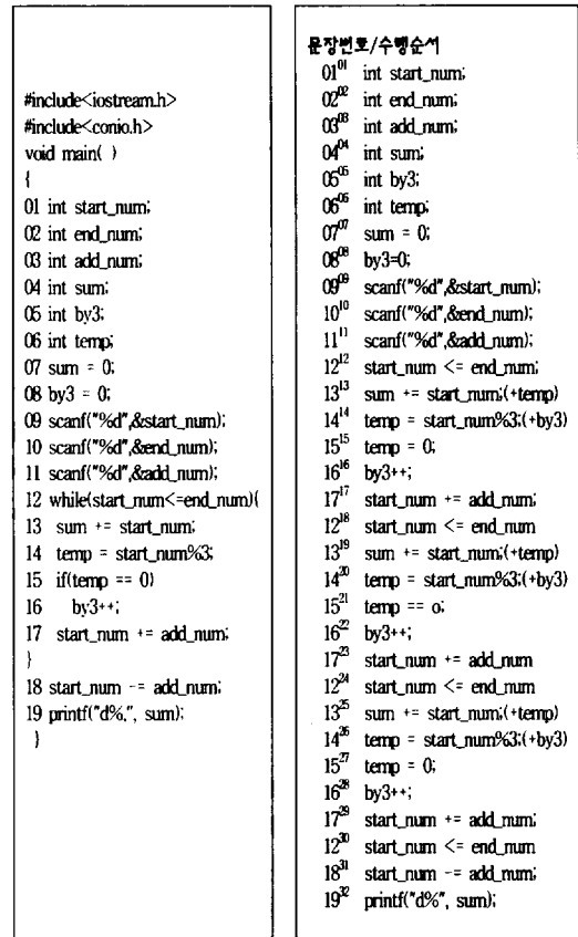
(a) 전체 프로그램(P) (b) 프로그램에 대한 수행 정보(T)
