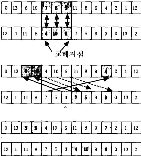
(그림 10) 교배연산 (Fig. 10) crossover operator
