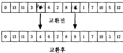
(그림 11) 돌연변이 연산 (Fig. 11) mutation operator
